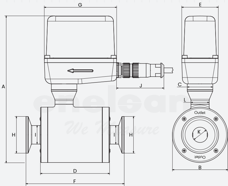
Emfil25 xx Dimensions (mm)
